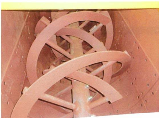
羽根形状
